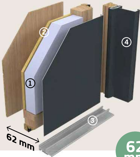
INTÉRIEUR BOIS
